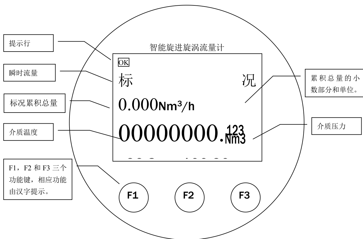
液晶显示屏图示
