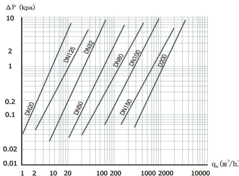
压力损失曲线
